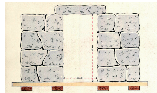
Eksempel på tørrmurt kloakk – her fra Lakkegata i Oslo.
